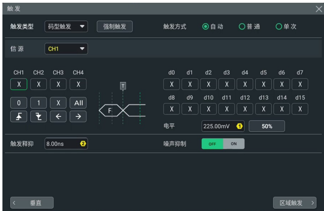
图 8.10 码型触发配置菜单
