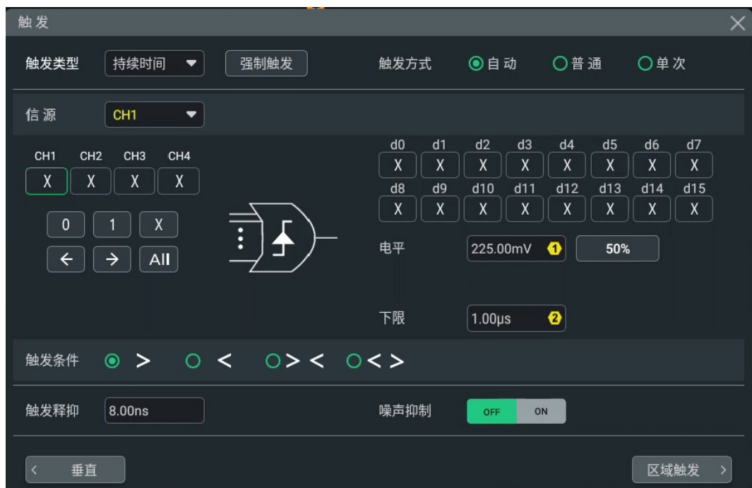
图 8.12 持续时间触发配置菜单
