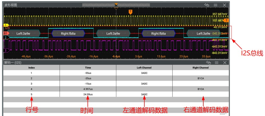
图 19.19 I2S 解码事件表
